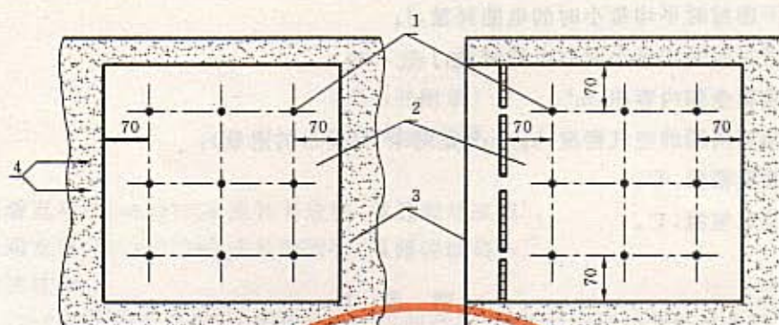
1—测定位置;2—透明板;3—开口处;4—风向
