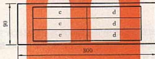
图 1 沥青基防水卷材取样图
