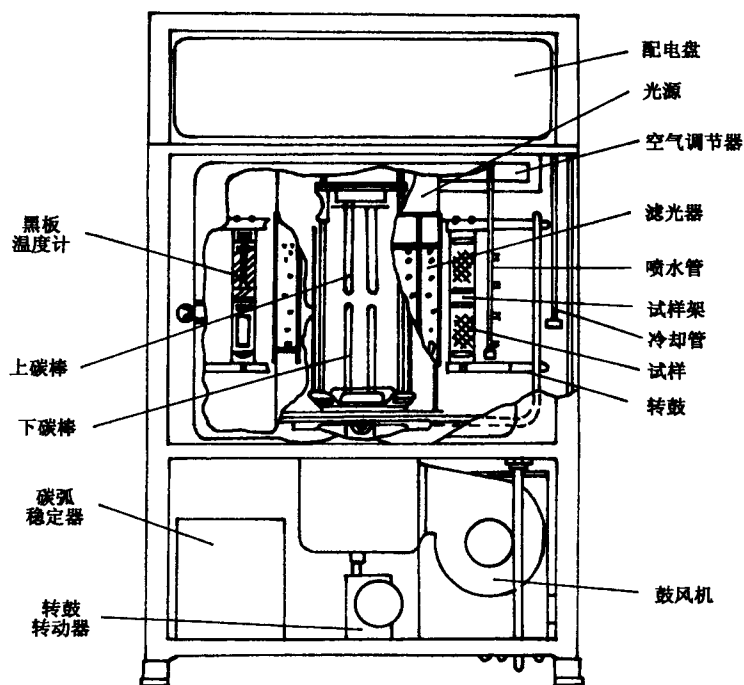
图 G1 碳弧灯试验箱
