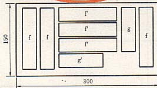
图 2 高分子防水卷材取样图
